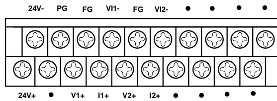
图 4-1 MC200-2AD 模拟量输入模块用户端子图
