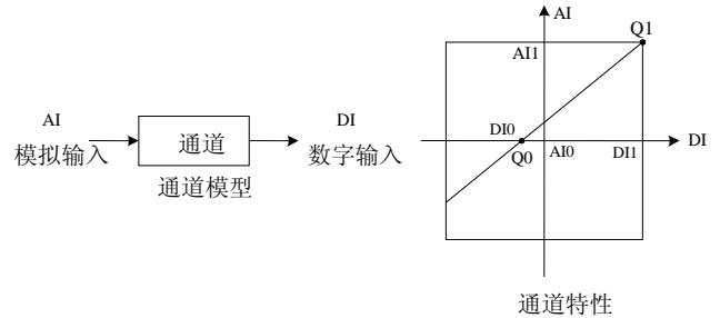
图 5-1 MC200-2AD 的通道特性示意图
